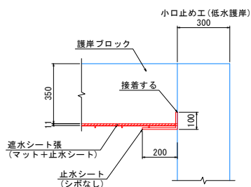
小口止め工接続部詳細図
