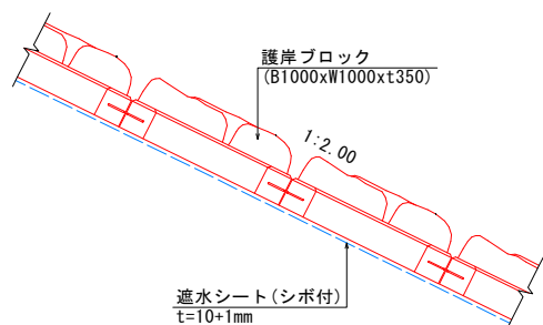
小口止め工接続部詳細図
