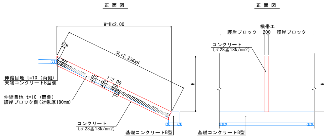
横帯工詳細図 S=1:50 (低水護岸工)
