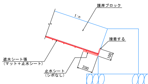
基礎コンクリート部詳細図
