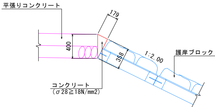
天端コンクリートB型 S=1:20 (低水護岸工)
